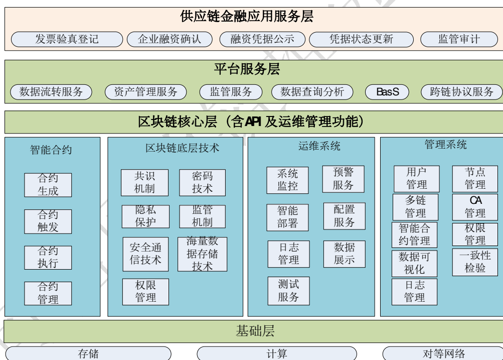
图7 航天信息区块链平台架构
